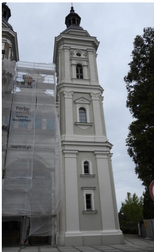
Zdjęcia 25 i 26 - Końcowy odbiór konserwatorski - Renowacja i konserwacja zabytku - kościoła p.w. św. Andrzeja Boboli w Krotoszynie –II etap (maj 2025).
