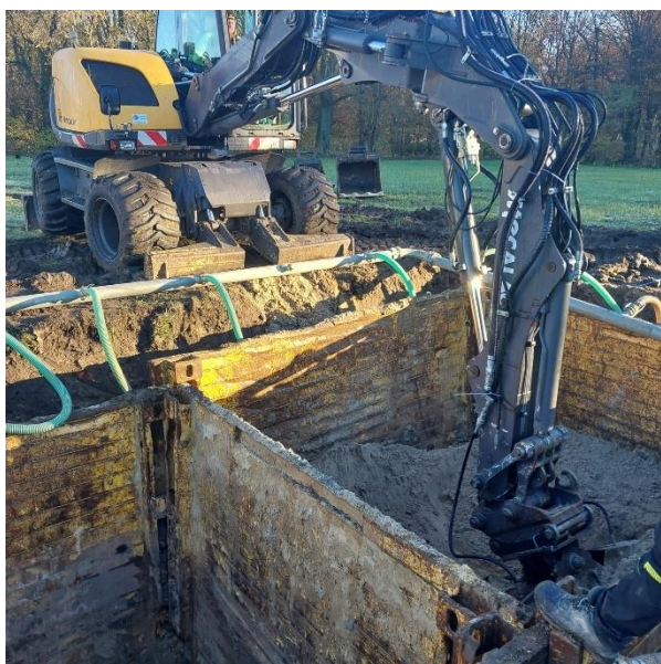
Zdjęcie 3. Prace przy montażu zbiorników na deszczówkę w DPS Baszków (wrzesień/październik).
